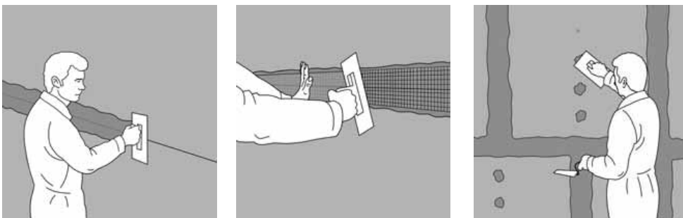
Рис. 14. Шпаклевание стыков и мест установки шурупов.
