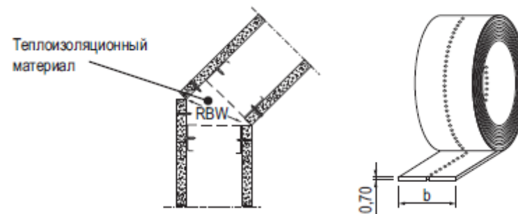
Рис 6. Соединение стеновых панелей под произвольным углом
