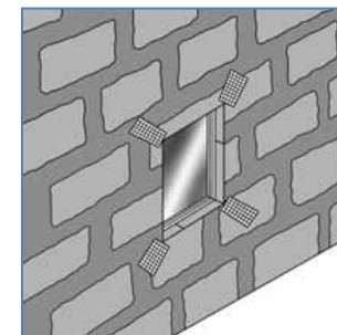
Рис. 19. Армирование обшивки в углах оконных и дверных проемов
