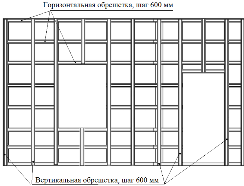
Рис. 5 Схема расположения вертикальной обрешетки
