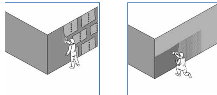
Рис. 20. Нанесение базового штукатурного слоя
