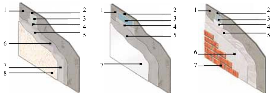
Рис. 15. Декоративное оштукатуривание наружной обшивки
