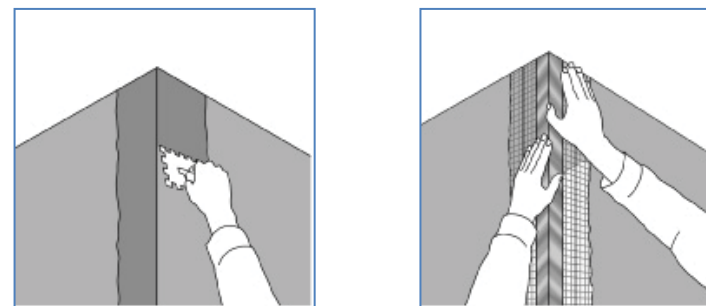
Рис. 18. Армирование углов
