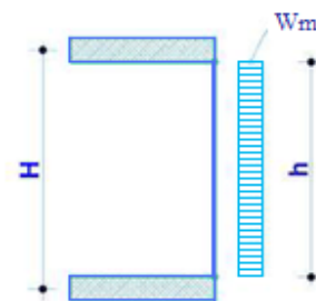
Рис. 3 Расчетная схема стойки каркаса стены при воздействии ветровой нагрузки
